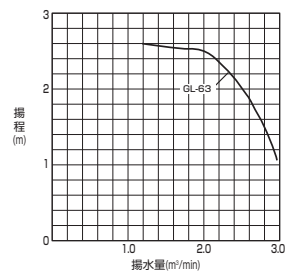
■性能曲線
