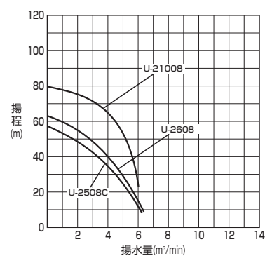
■性能曲線
